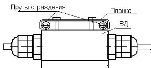
Рис.3.10. Способ установки ВД на сетчатых ограждениях
