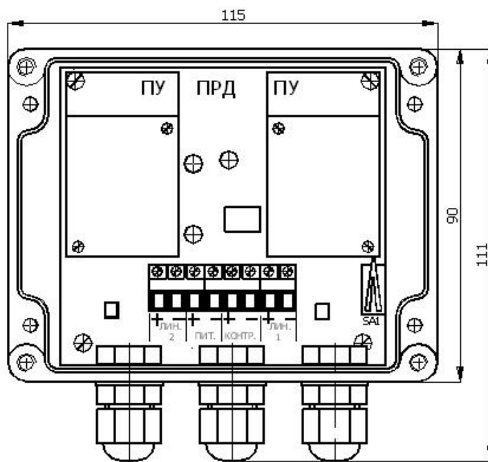
Рис.2.2 Общий вид ПРД
