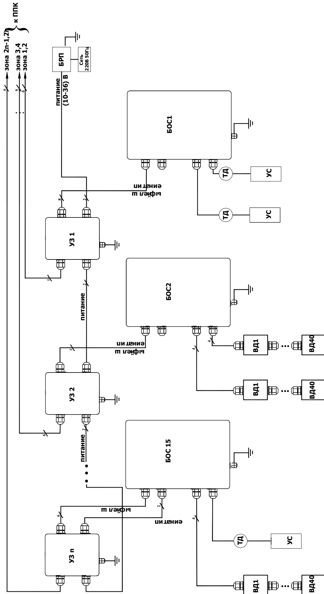
Рис.П.4. Схема соединений извещателей при непосредственной установке БАС, по периметру зоны охраны, с передачей извещений по шлейфам.
