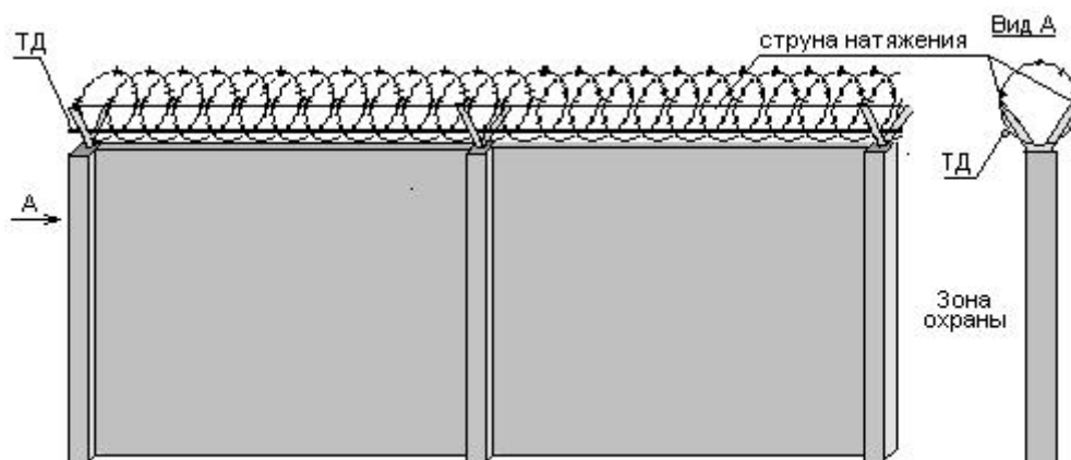
Рис.3.5. Способ прокладки ТД по козырьку из колючей проволоки
