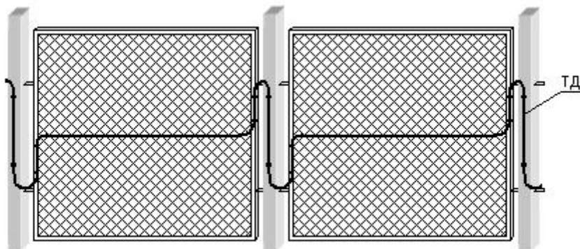
Рис.3.4. Способ прокладки ТД для секционных ограждений
