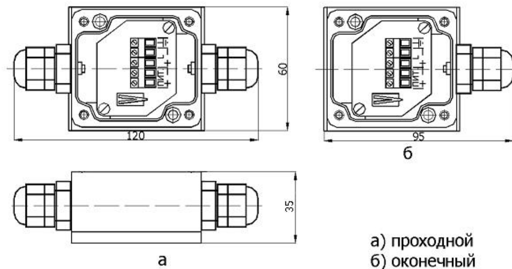
Рис.2.6 Общий вид ВД
