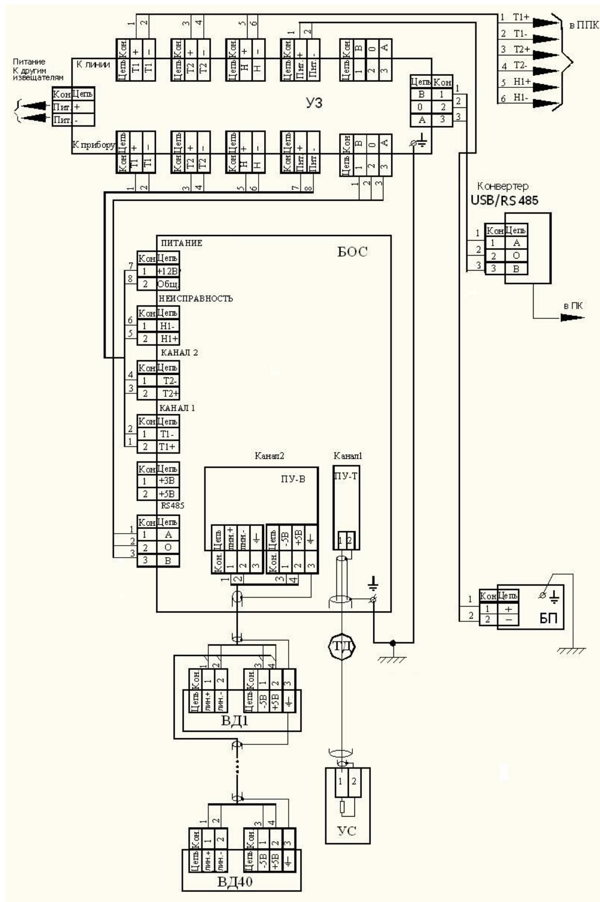
Рис. П.1. Схема подключения извещателя при непосредственной установке БОС
