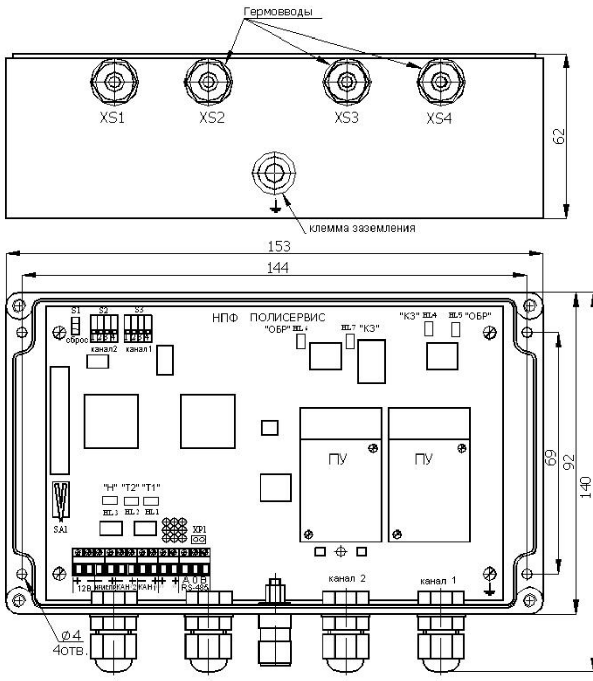
Рис.2.1 Общий вид БОС
