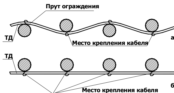
Рис.3.7. Способы крепления ТД к сетчатым ограждениям
