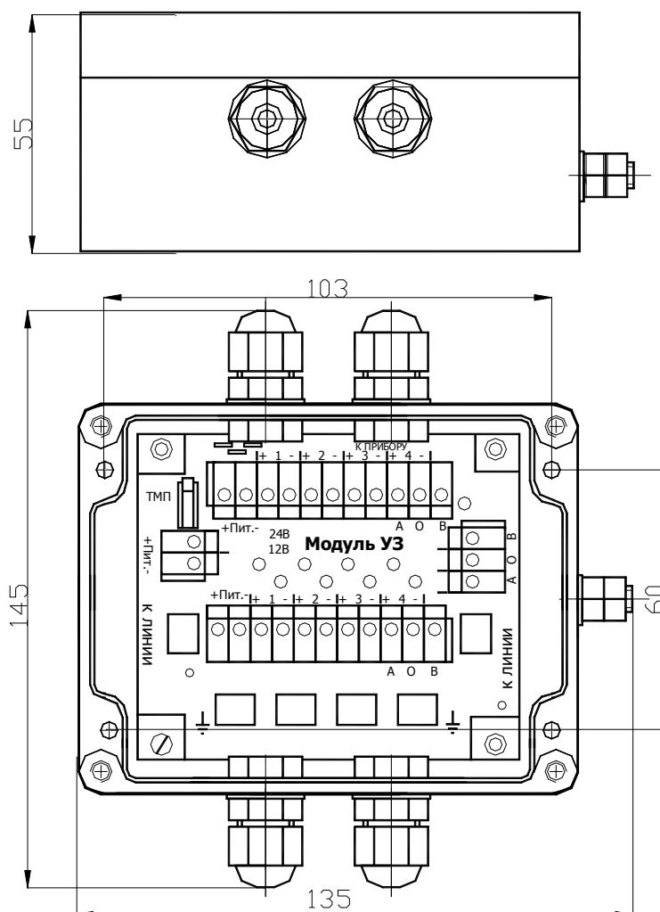
Рис.2.7 Общий вид УЗ
