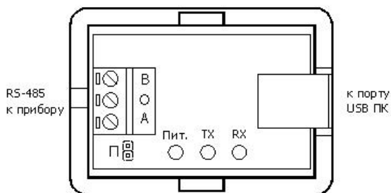
Рис.2.8. Общий вид конвертера со снятой крышкой
