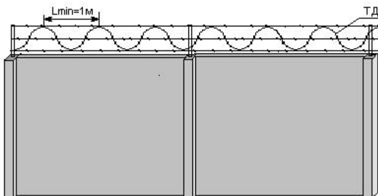
Рис.3.4. Способ прокладки ТД для секционных ограждений
