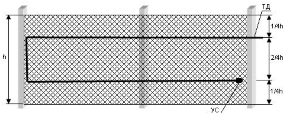
Рис.3.2. Способ прокладки ТД для жёстких ограждений
