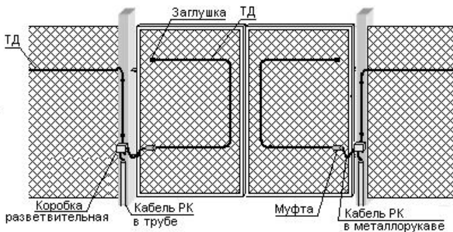
Рис.3.8. Способ оборудования ворот
