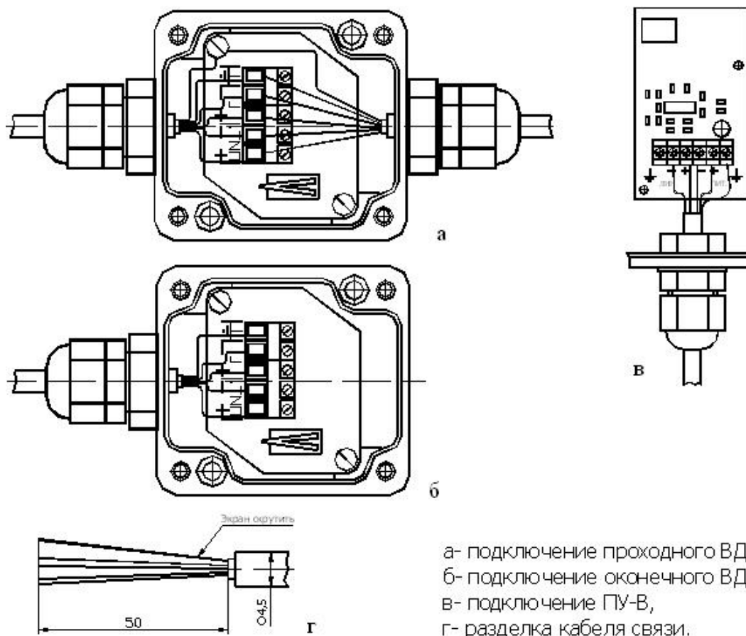
Рис.3.13. Подключение ВД
