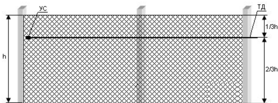
Рис.3.1. Способ прокладки ТД для мягких ограждений
