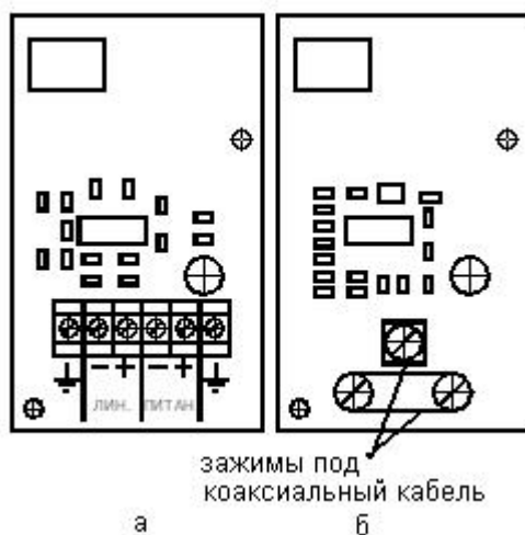
Рис.2.3 Общий вид ПУ а. – ПУ-В, б. – ПУ-Т (экран не показан)
