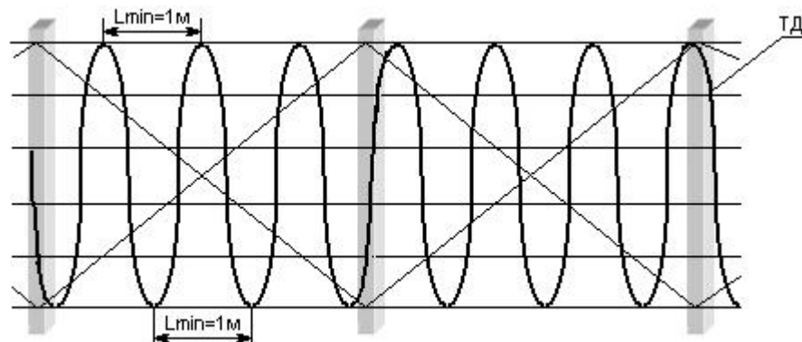
Рис.3.3. Способ прокладки ТД для ограждений из колючей проволоки
